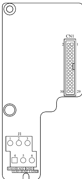
图 G-1 SEP-AI1 外形尺寸图
