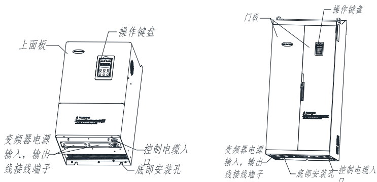
图 2-3 SEP200 系列变频器各部位名称示意图
