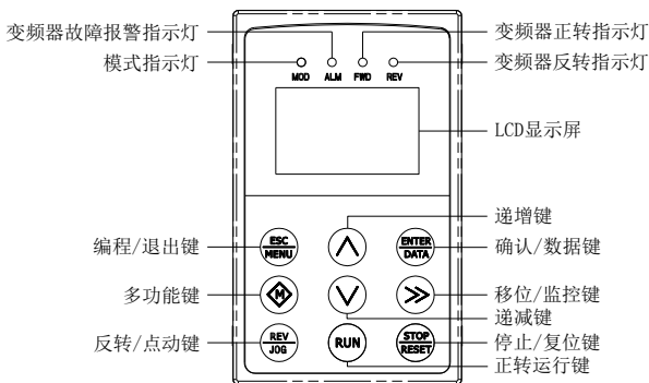
图 C-2 SEP-LCD1、SEP-LCD2 操作键盘布局图
