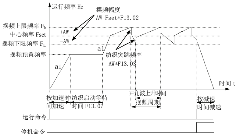
图 7-43 摆频示意图
