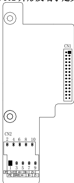
图 E-1 SEP-PG01、SEP-PG02 外形尺寸图
