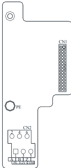
图 E-2 SEP-PG03 外形尺寸图
