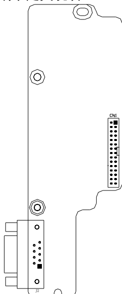
图 E-3 SEP-PG04 外形尺寸图
