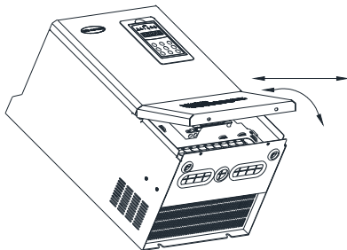
图 3-5 钣金盖板的拆卸与安装图
