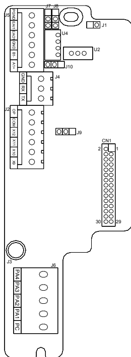
图 H-1 SEP-PLC1 外形图
