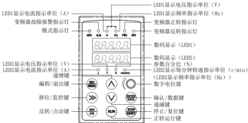
图 C-1 SEP-LED4-D 操作键盘布局图
