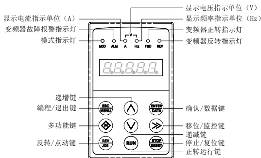
图 C-8 SEP-LED1 操作键盘布局图
